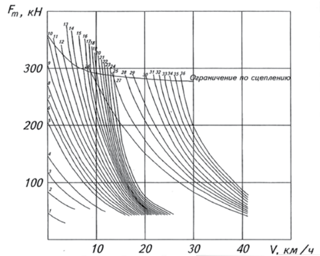
Тяговые характеристики тягового агрегата ПЭ-2М
