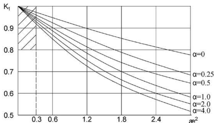
Рис. 5. Зависимость коэффициента K_1 от параметров \alpha и ae^2 (заштрихована зона, в пределах которой допускается пренебрежение упругостью)
