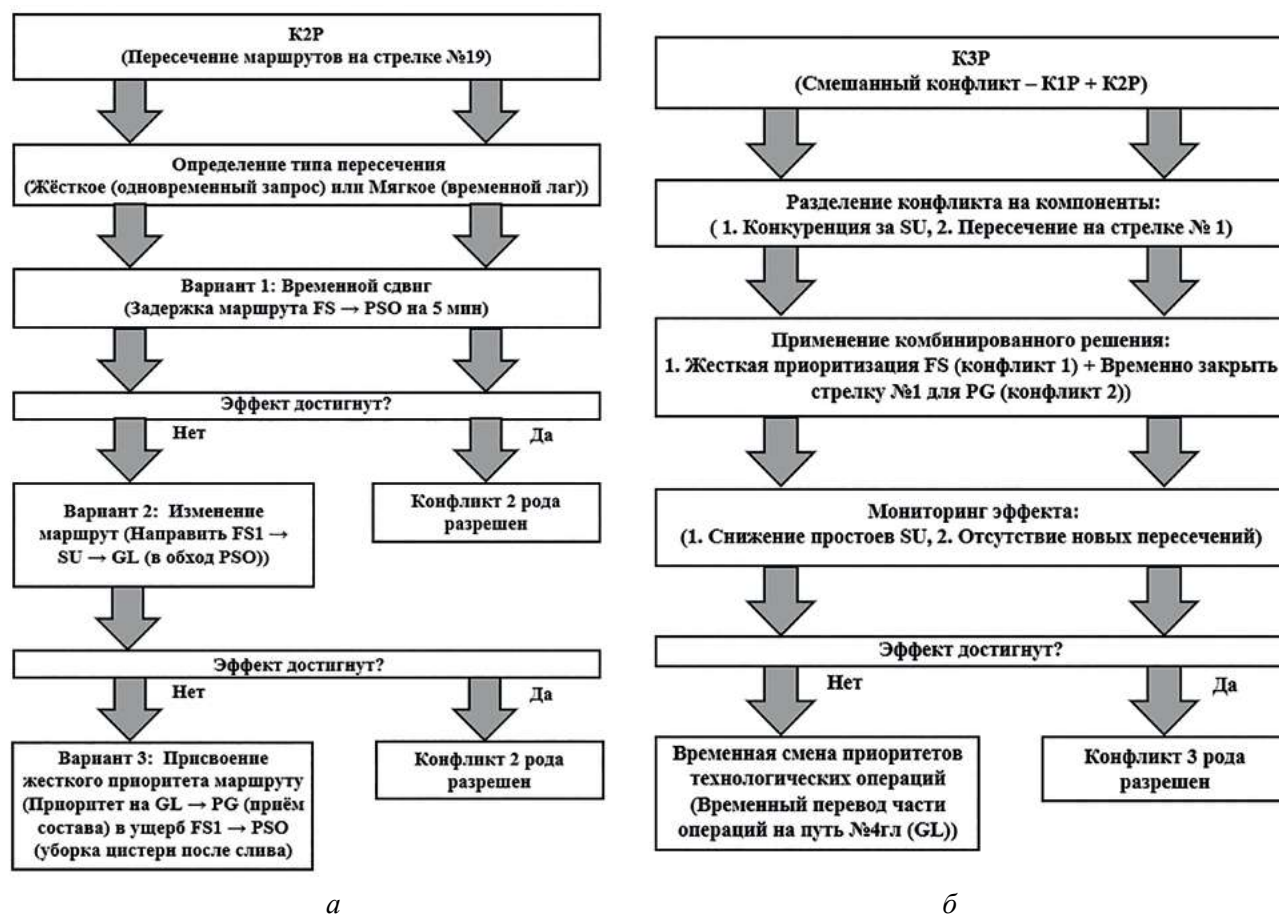
Рис. 7. Укрупненные блок-схемы решения транспортных конфликтов по вариантам управления местной работой станции «Г»: а — K2P, б — K3P
