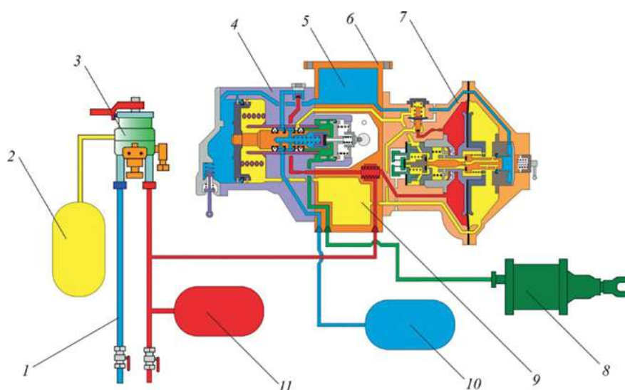
Рис. 4. Пневматическая схема станда для проверки работы воздухораспределителя грузового типа:
