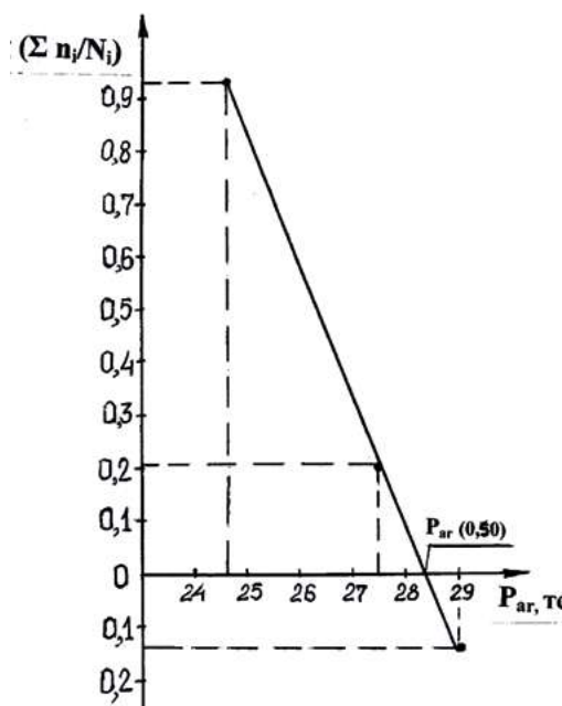
Рис. 8. Графическое определение предела выносливости боковых рам тележки модели 18-9891 (черт. № 9891.01.00.001) по результатам испытаний методом Локати (II режим нагружения)
