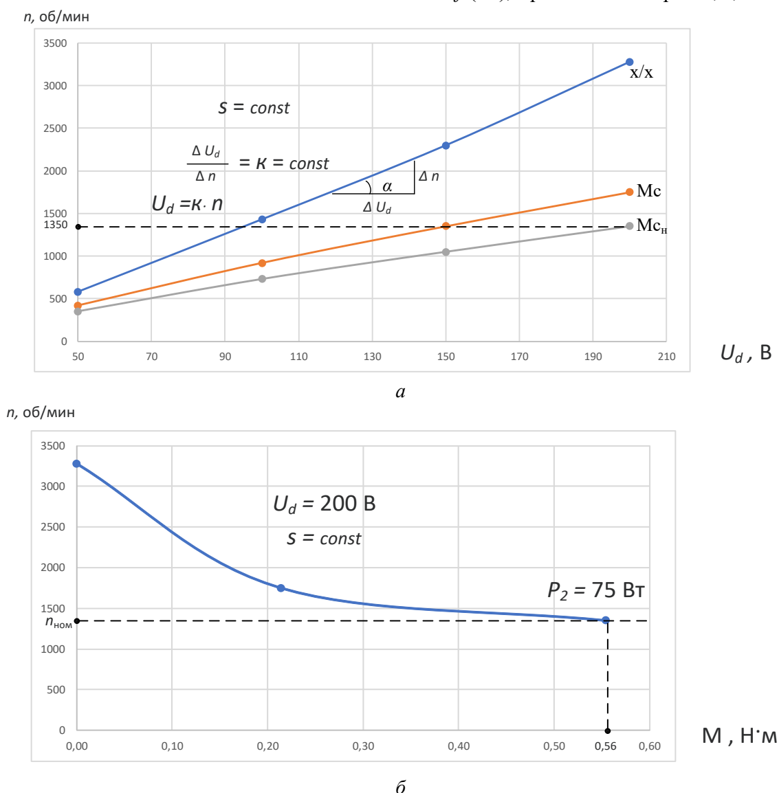
Рис. 6. Характеристики привода: а — регулировочная, б — механическая
