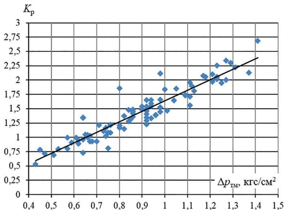
Рис. 6. Определение коэффициента влияния степени торможения на время отпуска тормозных цилиндров грузовых вагонов: \Delta p_{\text{тм}} — степень торможения, кгс/см 2
