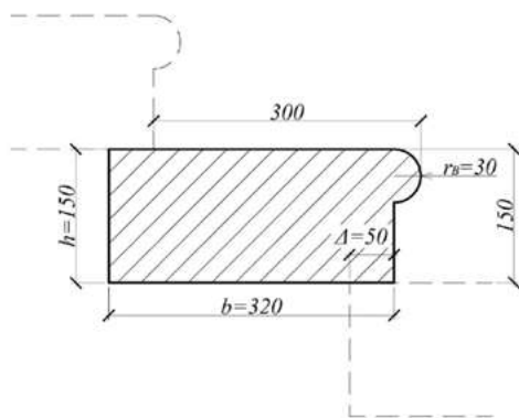
Рис. 3. Сечение ступени
