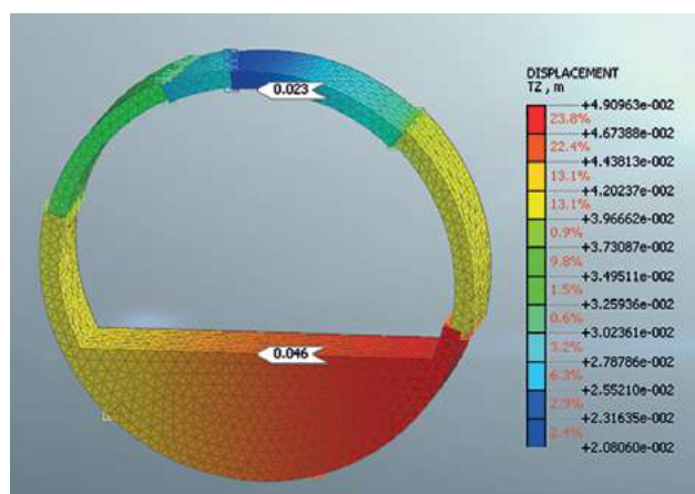
Рис. 7. Расчет № 3: изополя вертикальных деформаций обделки
