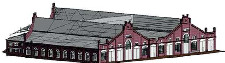
Рис. 2. Построенная BIM-модель бывшего вагоностроительного завода им. И. Е. Егорова [7]
