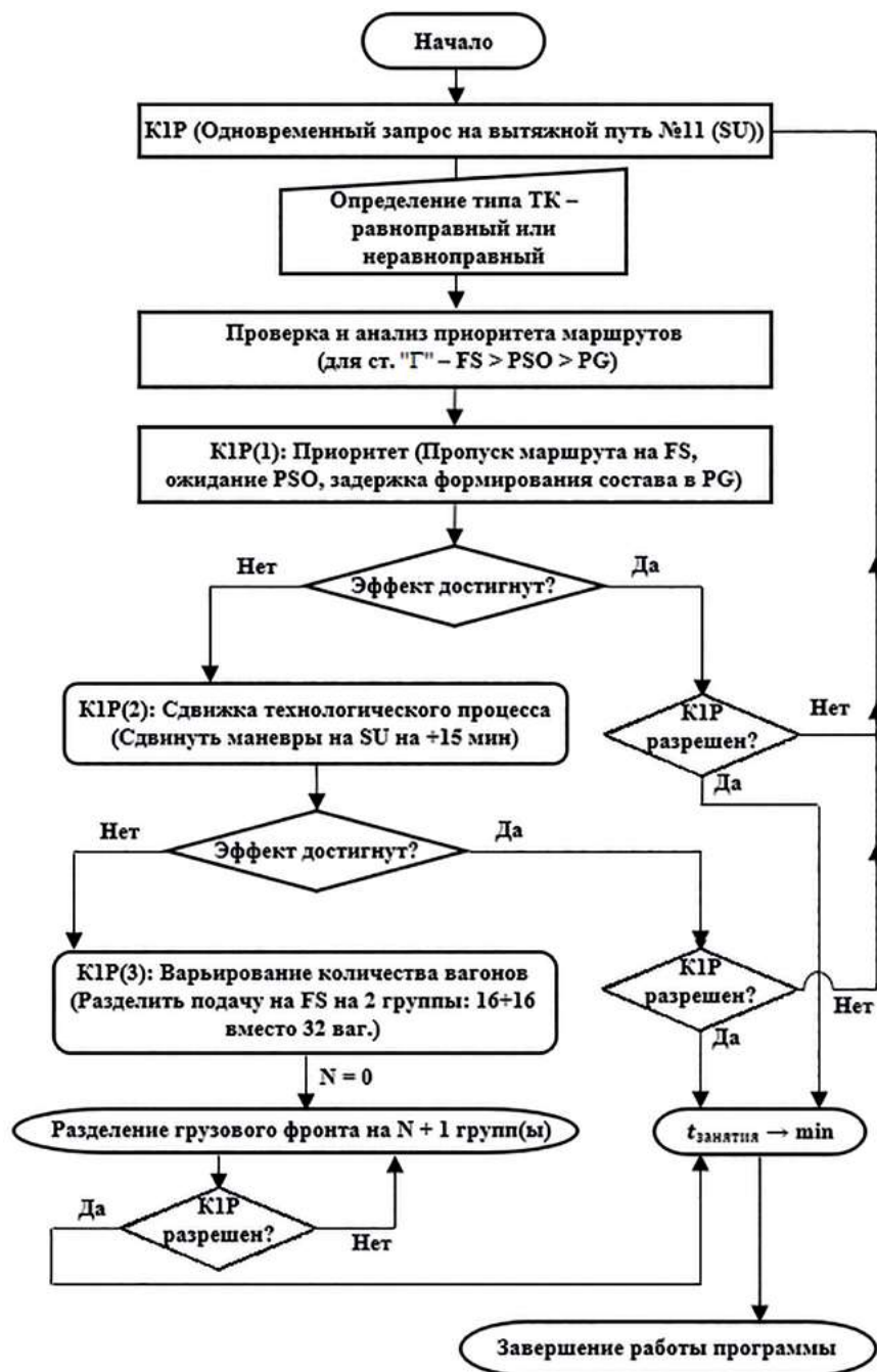
Рис. 6. Блок-схема решения K1P по варианту транспортной работы припортовой станции «Г»
