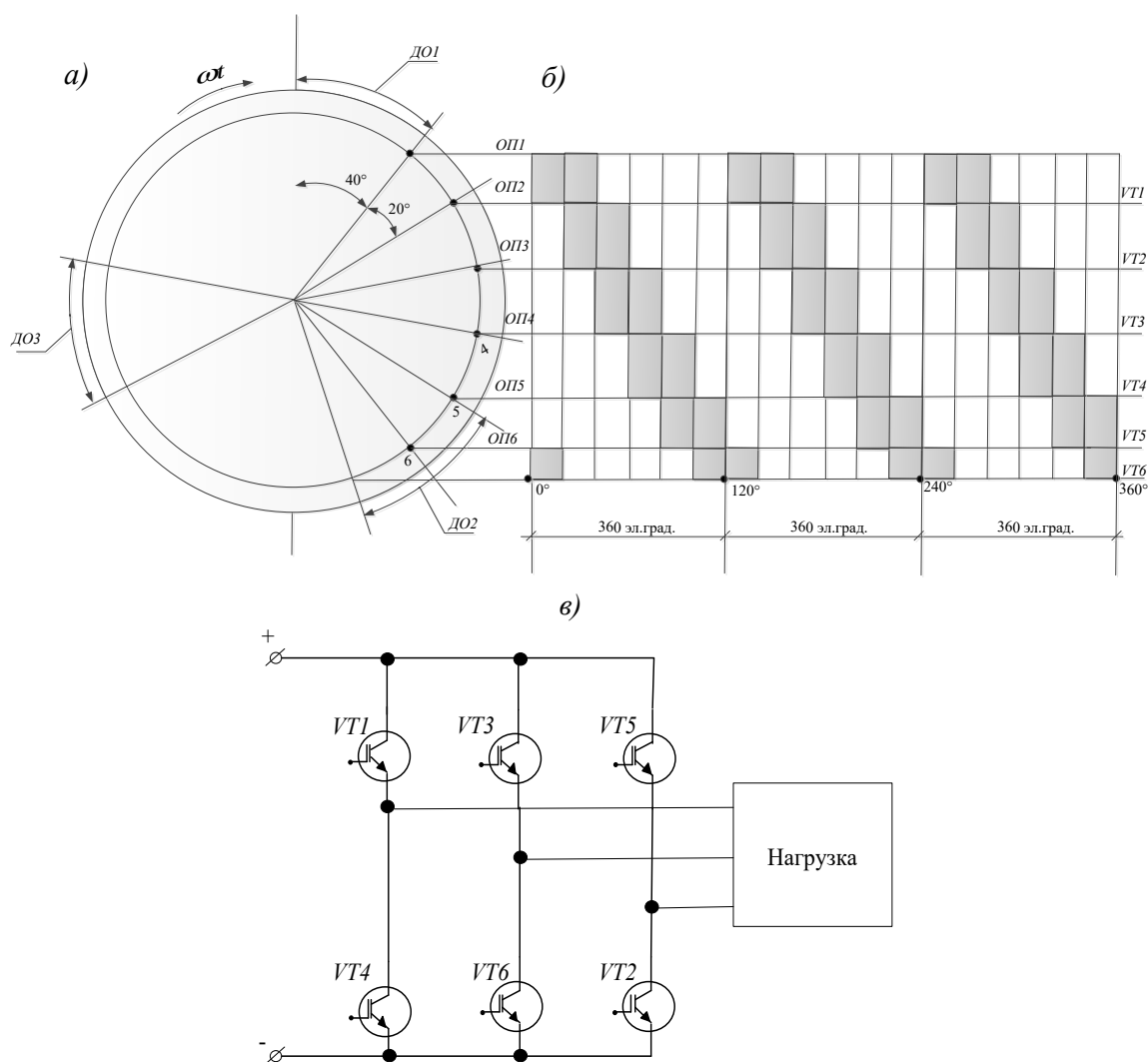
Рис. 2. Формирование алгоритма:
